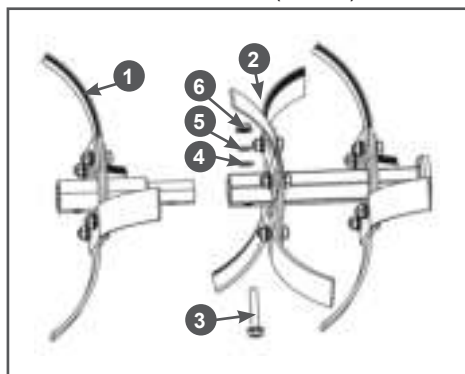
Рис. 9 Соединение основной и дополнительной секций фрезы 1. Секция фрезы дополнительная 2. Секция фрезы основная 3. Болт 4. Шайба плоская 5. Шайба пружинная 6. Гайка
