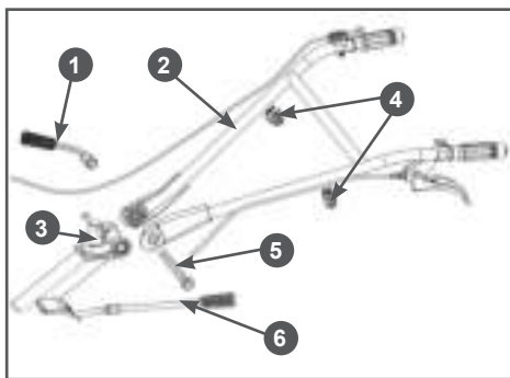
Рис. 14 Установка рабочих рукояток
