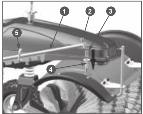
Рис. 3 Установка рычага управления поворотом щетки
