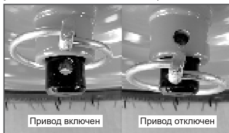
Рис. 17 Перестановка шплинта на левом колесе
