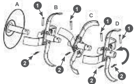
Рис. 3 Установка фрез
