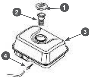
Рис. 21 Топливные фильтры
