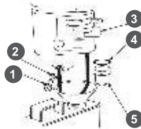
Рис. 23 Обслуживание фильтра-отстойника
