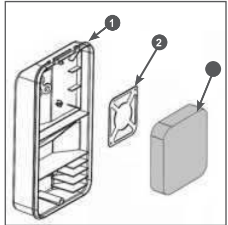
Рис. 1 Обслуживание воздушного фильтра
