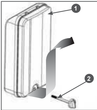
Рис. 1 Снятие крышки воздушного фильтра
