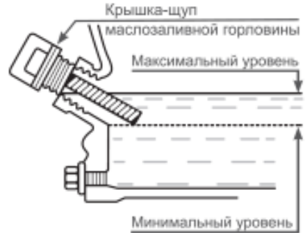
Рис. Проверка уровня масла в картере
