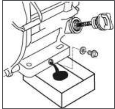
Рис. 1 Замена масла в двигателе
