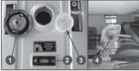
Рис.1 Основные элементы топливного бака
