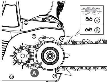
Рис. 3 Установка шины А - Колесо накладке шины
