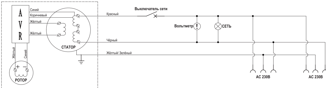
ГЕНЕРАТОР ПЕРЕМЕННОГО ТОКА
