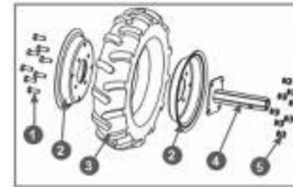
Рис. 15 Сборка колеса
