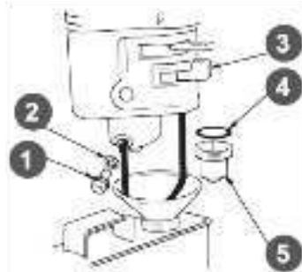
Рис. 21 Обслуживание фильтра-отстойника
