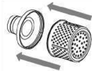
Рис. 9 Сборка всасывающего фильтра
