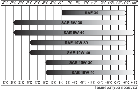
Рис. 7 Определение вязкости масла
