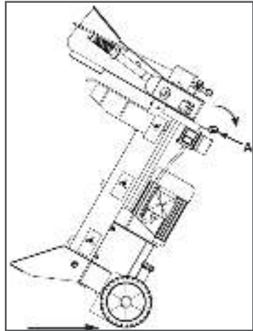
Рис. 12 Перемещение дровокола
