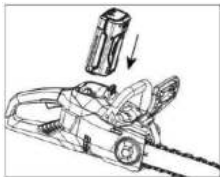
Рис. 6. Установка аккумулятора
