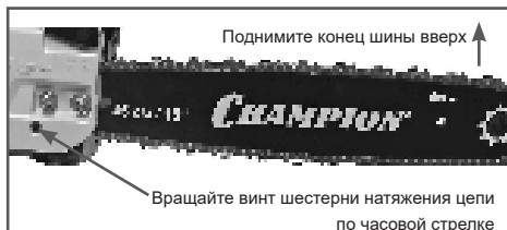
Рис. 5 Регулировка натяжения цепи
