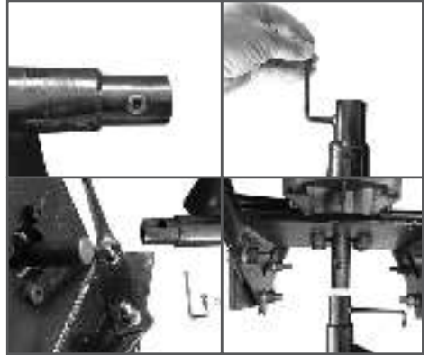
Рис. 3 Установка шнека на мотобур
