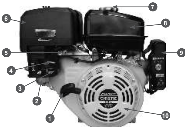
Рис. 3 Основные узлы и органы управления двигателя (вид со стороны стартера)
