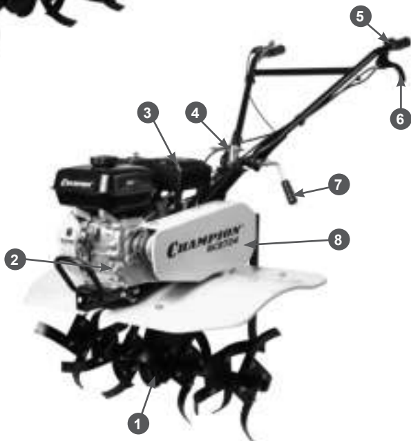
Рис. 2 Основные узлы и органы управления (вид слева)
