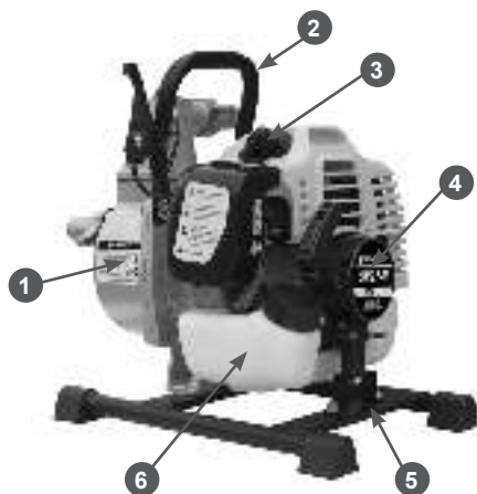
Рис.2 Расположение основных узлов и органов управления (вид сзади)
