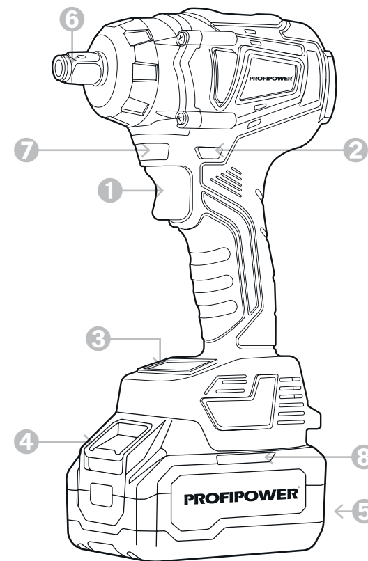
Рисунок 1.4.1. Устройство инструмента
