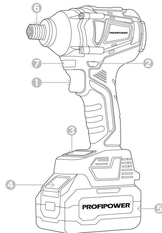
Рисунок 1.4.1. Устройство инструмента
