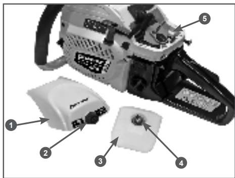
Рис. 21 Обслуживание воздушного фильтра
