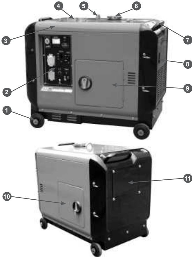
Рис. 1 Основные узлы и органы управления
