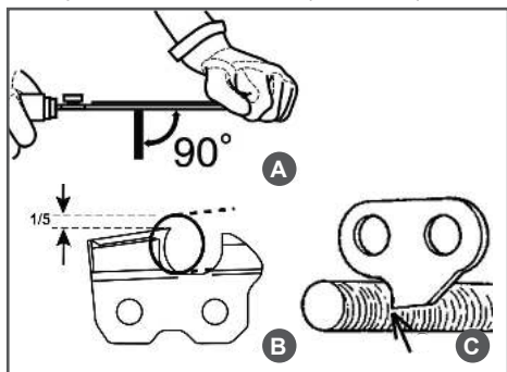
Рис. 30 Положение напильника при заточке
