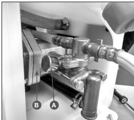
Рис. 13 Насос
