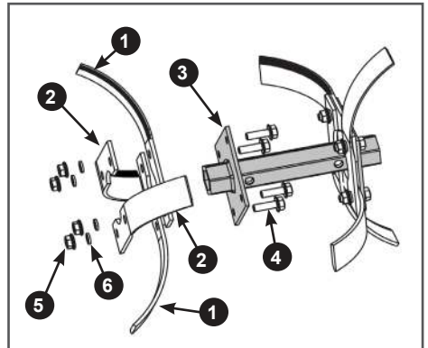
Рис. 18. Установка ножей на внутренний фланец основной секции оси фрезы
