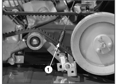
Рис. 42. Пружина троса включения хода
