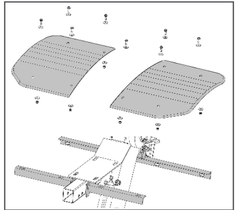
Рис. 9. Установка защитных крыльев
