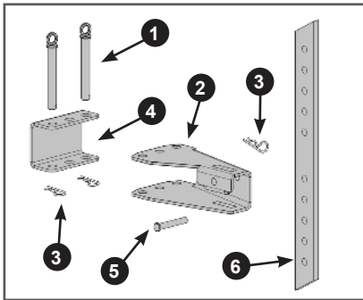
Рис. 7. Установка сошника
