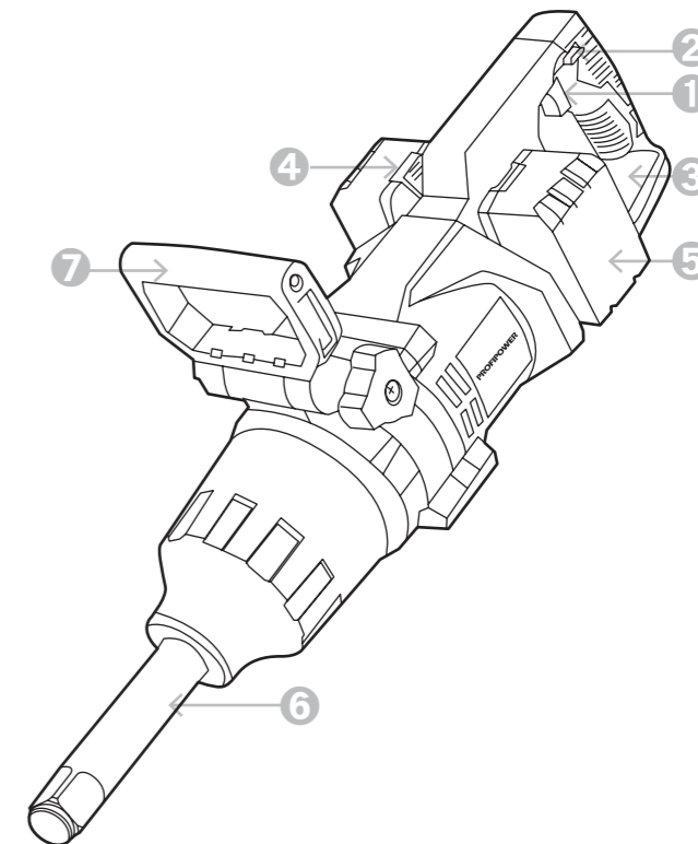
Рисунок 1.4.1. Устройство инструмента
