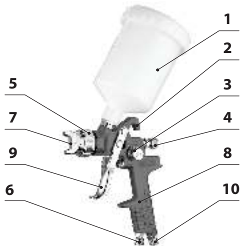
Внешний вид модели HVLP 1.4A (Рис. 3)
