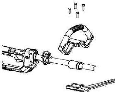
Рис. 4 Установка рукояток
