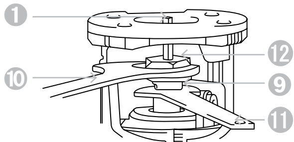
Рисунок 2.2.1. Установка фрезы
