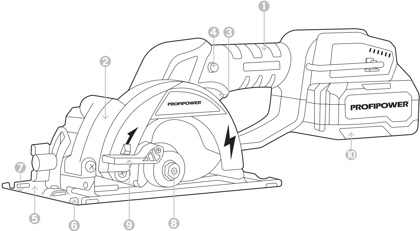
Рисунок 1.4.1. Устройство инструмента
