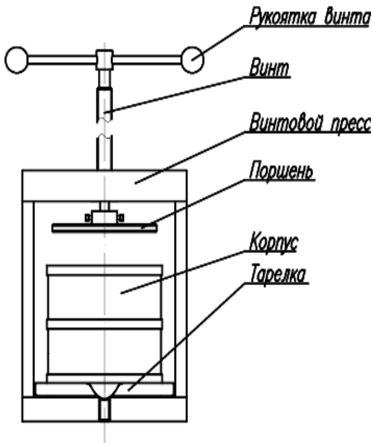
Рис. 1 Устройство изделия
