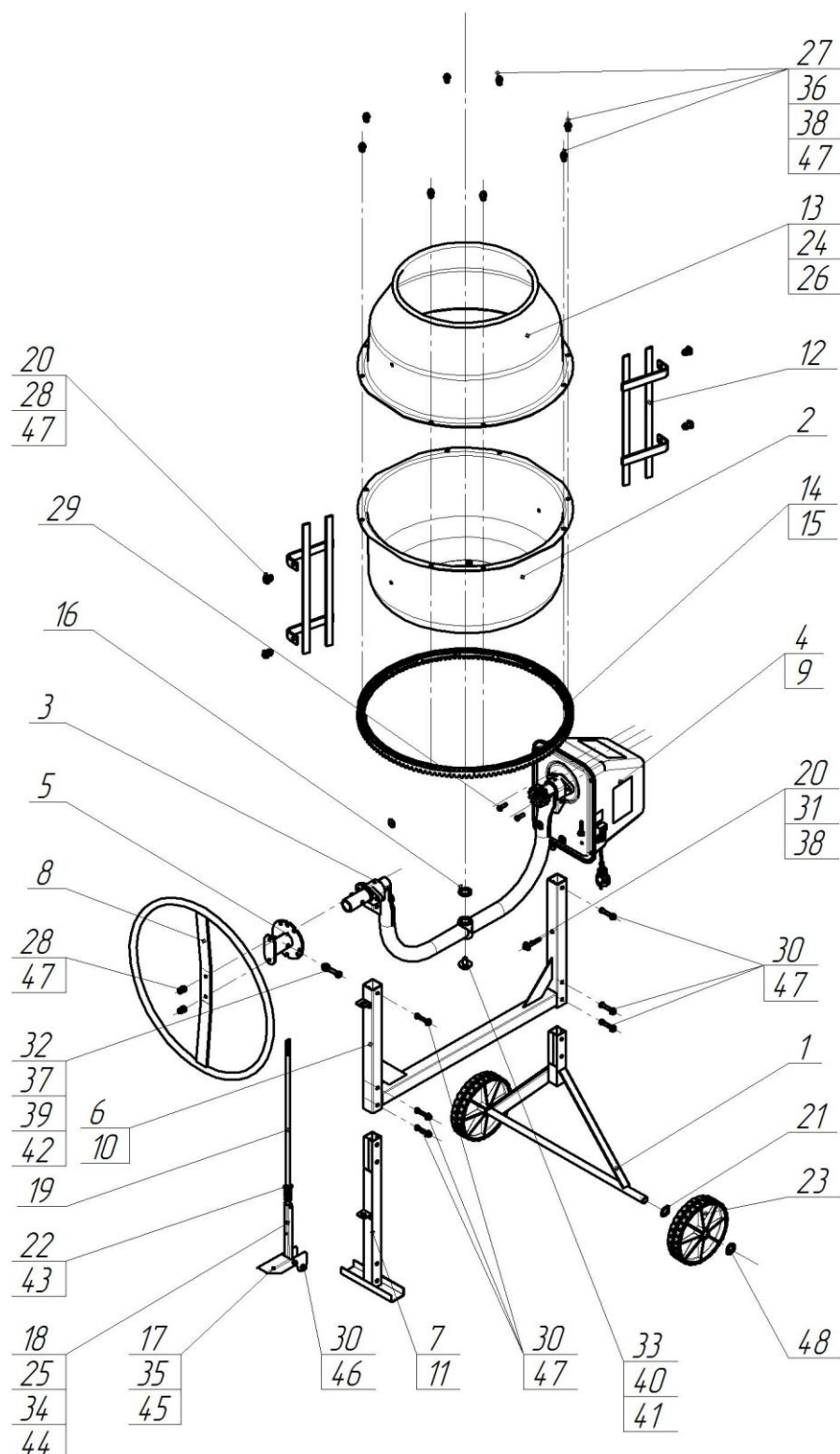
Схема – состав бетоносмесителя
