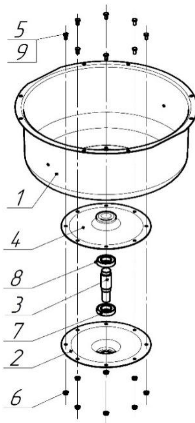
Схема-состав емкости нижней в сборе
