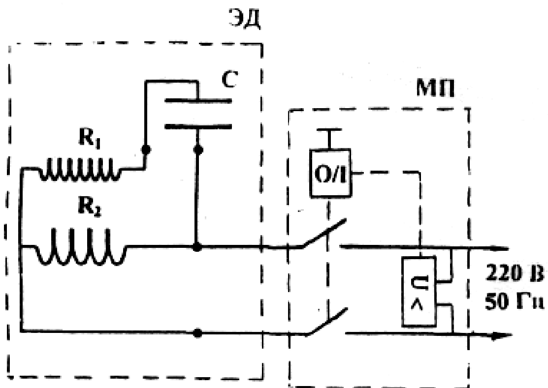
ЭД – электродвигатель, МП – магнитный пускатель.
