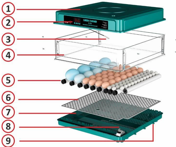
Рис. 1. Устройство инкубатора.
