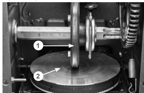
Рис. 41. Обслуживание трансмиссии
