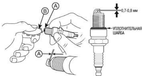
Рис. 38. Проверка межэлектродного зазора
