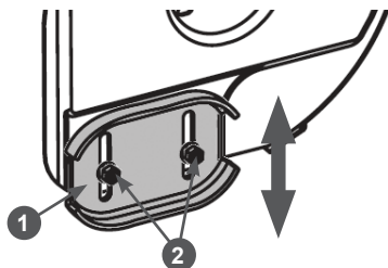
Рис. 25. Регулировка высоты забора снега 1. Ползочек 2. Гайка (2 шт.)
