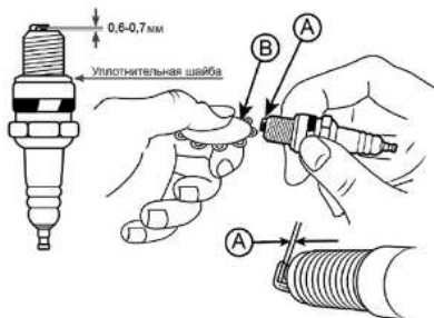
Рис. 32. Проверка зазора между электродами
