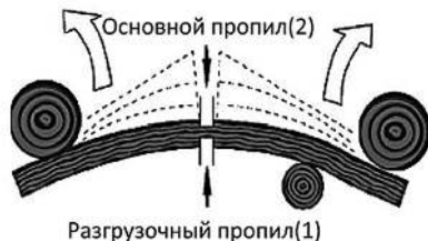
Рис. 27. Распиливание дерева, когда оба конца дерева зажаты и находятся под напряжением
