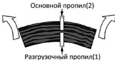
Рис. 24. Распиливание дерева, когда его верхняя часть находится под напряжением
