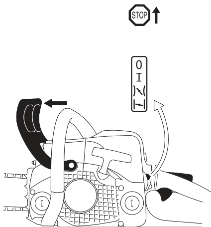
Рис.12. Положение комбинированного рычага при запуске
