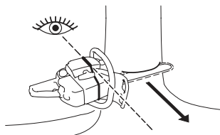
Рис. 22. Использование валовой планки
