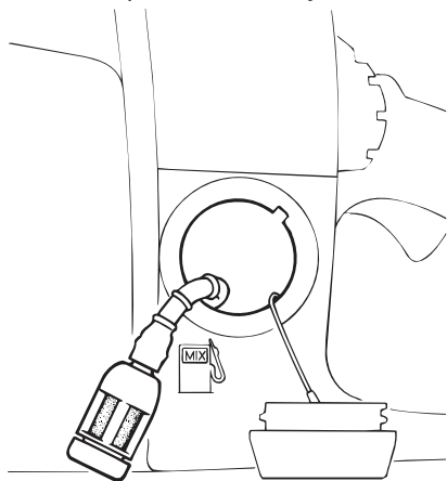
Рис. 30. Топливный фильтр
