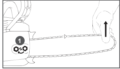
Рис. 6. Натяжение цепи
