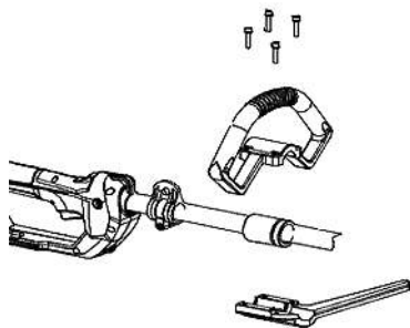
Рис. 4 Установка рукояток
