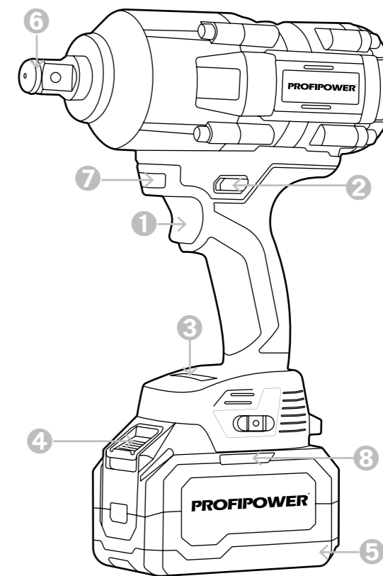
Рисунок 1.4.1. Устройство инструмента
