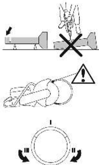
Рис. 15 Резка труб
