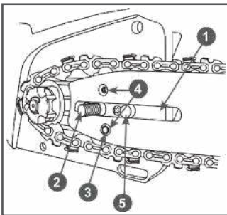
Рис. 4 Установка шины
