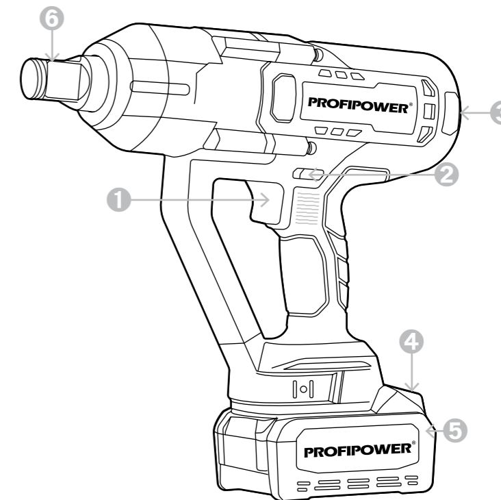
Рисунок 1.1. Устройство инструмента
