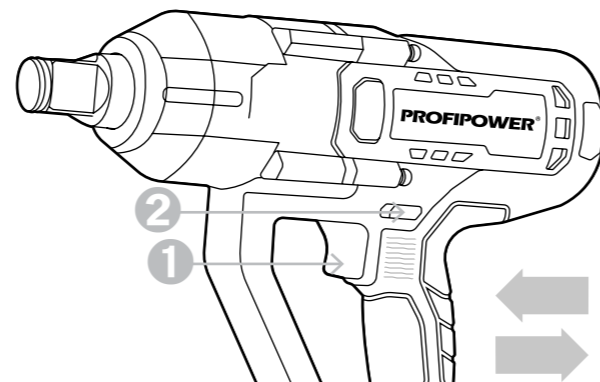
Рисунок 2.3.2. Установка направления вращения
