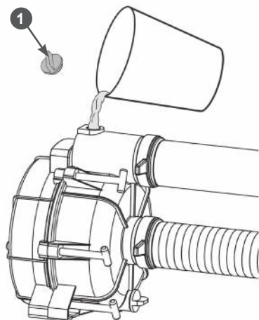
Рис. 13. Заполнение корпуса насоса водой 1. Пробка отверстия для заливки воды
