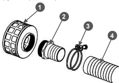
Рис. 10. Установка всасывающего фильтра
