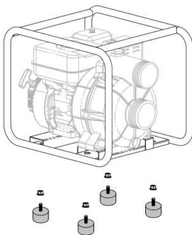
Рис. 5. Установка опор рамы
