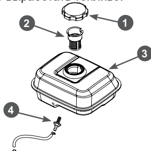
Рис. 23. Обслуживание топливных фильтров
