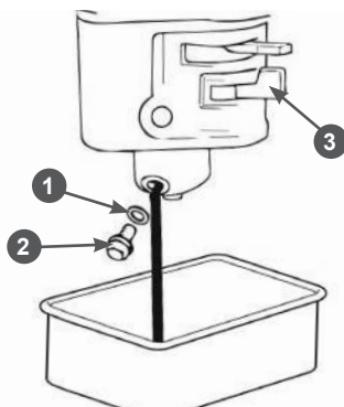
Рис. 25. Обслуживание карбюратора
