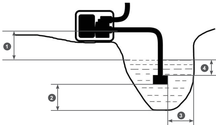
Рис. 12. Расположение мотопомпы и всасывающего фильтра
