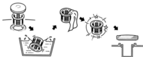
Рис. 24. Обслуживание фильтра топливного бака
