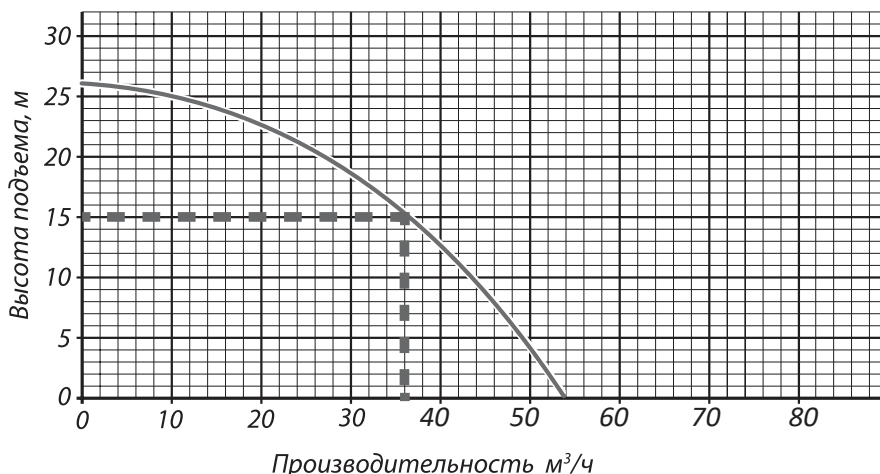
Рис. 28. График зависимости производительности мотопомпы от высоты подъема
