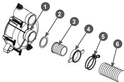
Рис. 11. Установка всасывающего рукава
