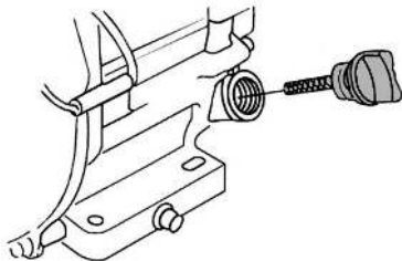
Рис. 7. Крышка-щуп маслозаливной горловины
