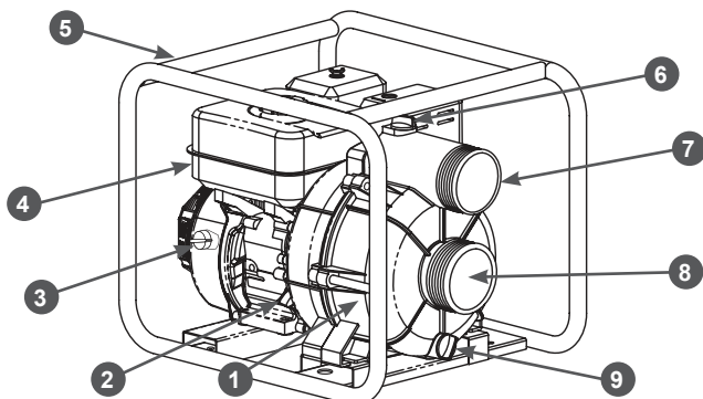
Рис. 2. Основные узлы и органы управления (общий вид)
