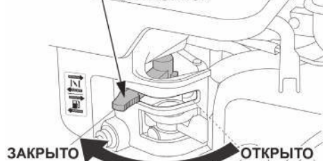
Рис. 14. Рычаг управления воздушной заслонкой
