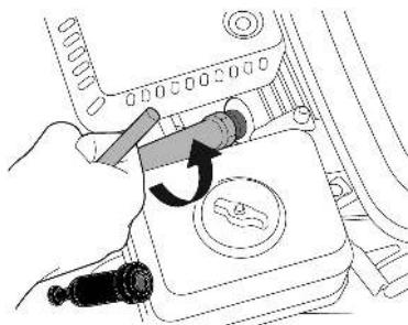
Рис. 26. Обслуживание свечи зажигания
