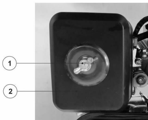
Рис. 13. Воздушный фильтр.
