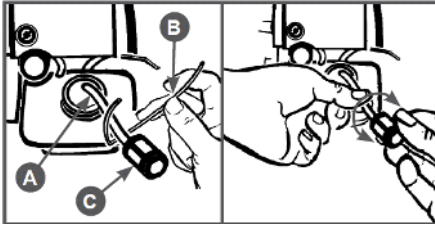
Рис. 14 Извлечение топливного фильтра
