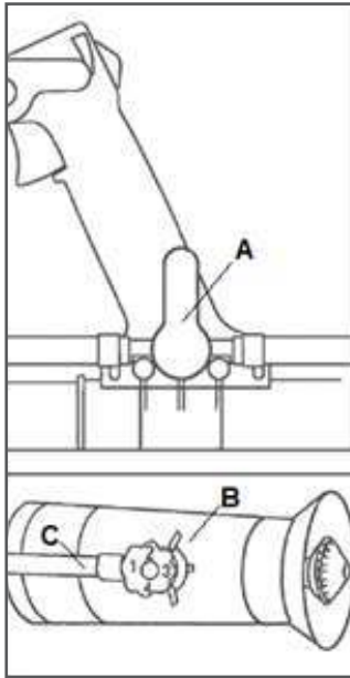
Рис. 11 Настройка дозатора
