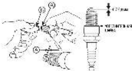
Рис. 41 Проверка межэлектродного зазора А- зазор В- щуп
