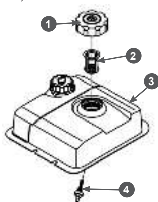
Рис. 38 Топливные фильтры
