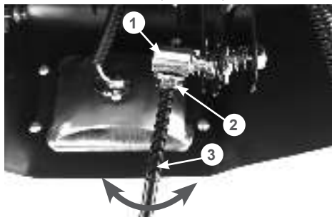
Рис. 17 Регулировка длины тяги рычага переключения передач
