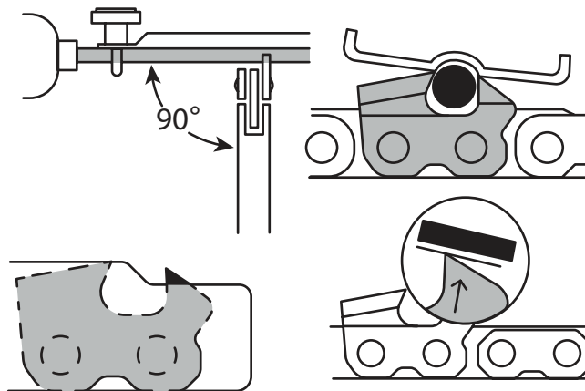
Рисунок 3.3.1. Заточка цепи
