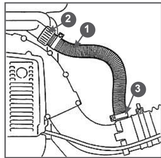
Рис. 10 Установка шланга распылителя
