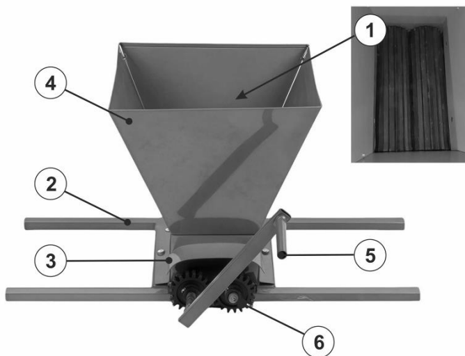
Рис. 1. Устройство моделей ДР-1, ДР-2.
