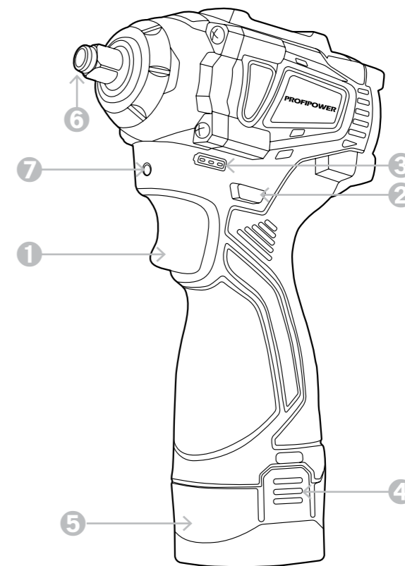
Рисунок 1.1. Устройство инструмента
