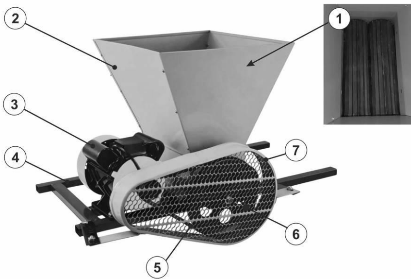
Рис. 1. Устройство модели ДЭ-1.
