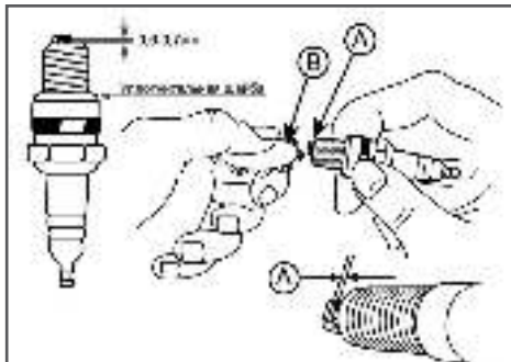
Рис. 21 Проверка зазора между электродами
