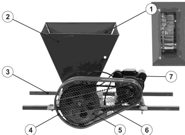
Рис. 1. Устройство модели ДЭ-2.
